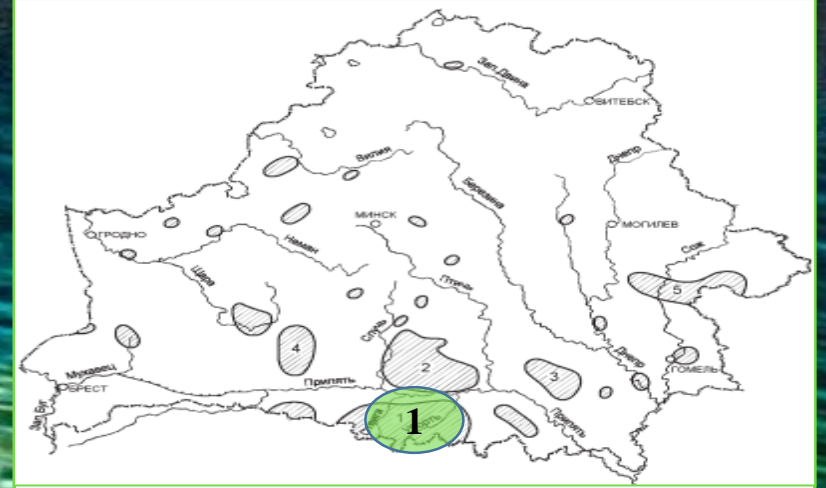
Наиболее крупная «линза» ультрапресных вод: 1 – Ствига-Убортская
